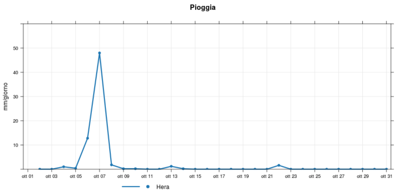
Figura 11: Pioggia cumulata nell'arco delle 24 ore
