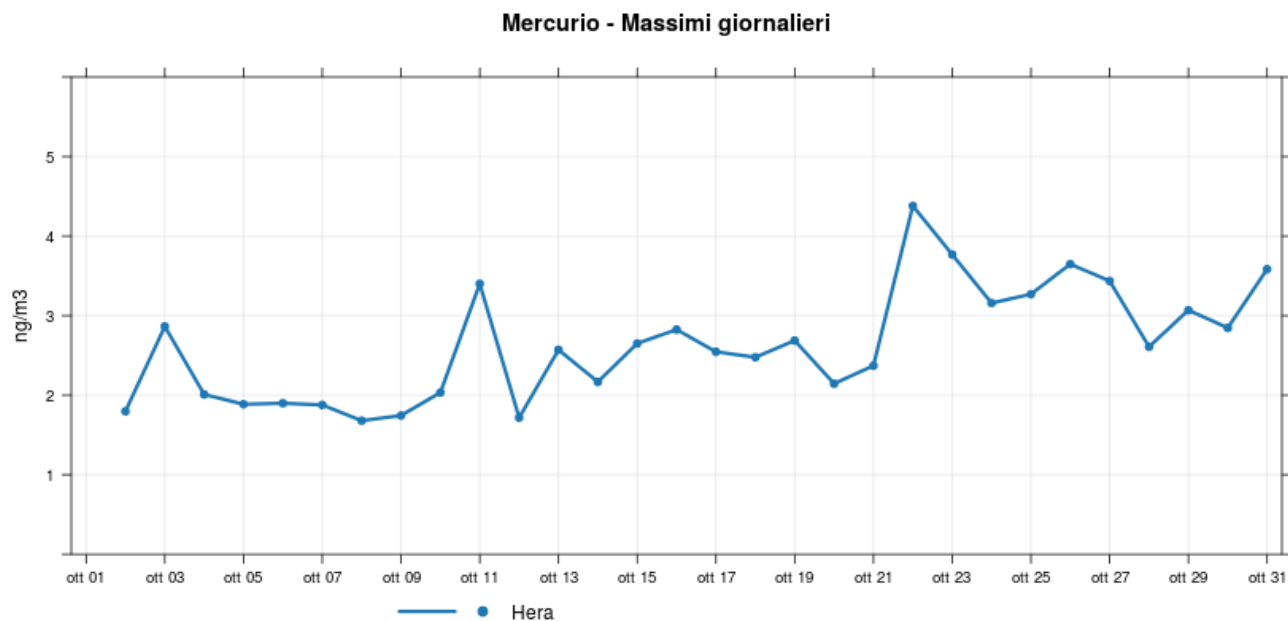
Figura 6: Massimi giornalieri di mercurio.
