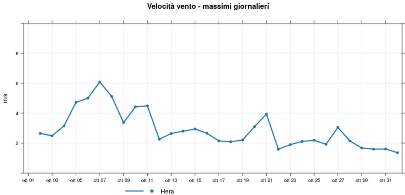
Figura 8: Velocità del vento – Massimi giornalieri
